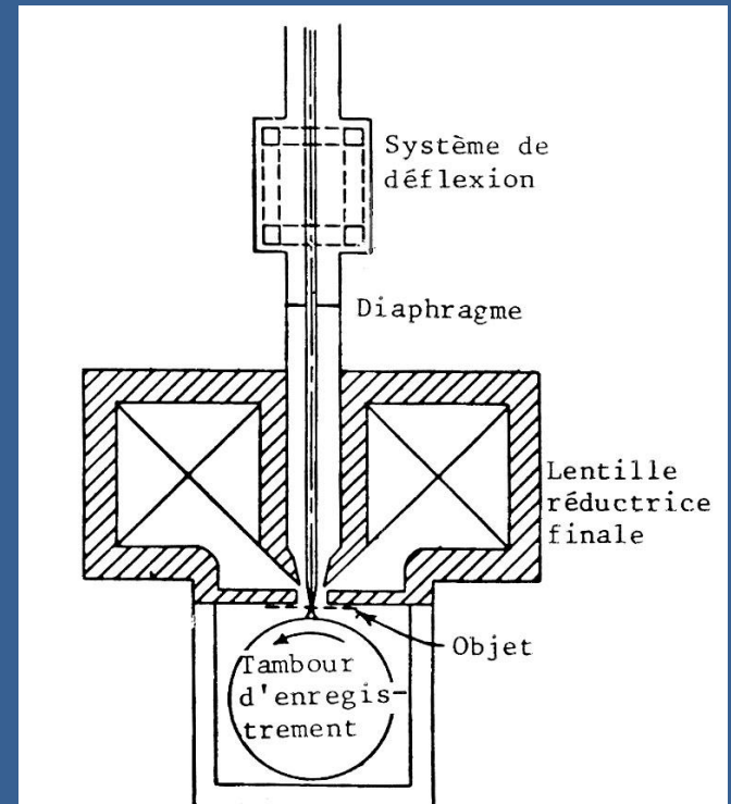
Le Microscope Electronique à Balayage de Von Ardenne (1938)
